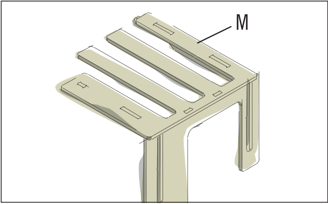
Monte le panneau de recouvrement à lattes (M) sur la partie inférieure montée précédemment.
