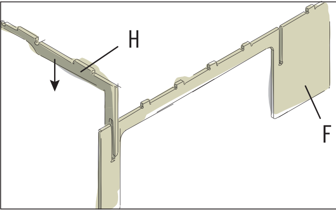
Emboîte le premier étau coudé (H) dans la fente gauche de la façade (F).
