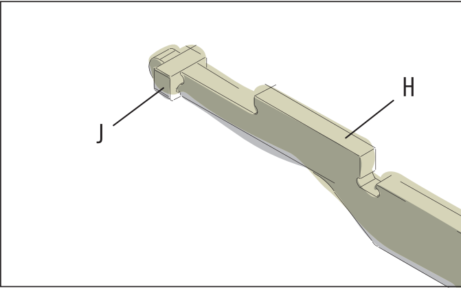
Le butoir empêche l'élément gigogne de sortir du cadre.
