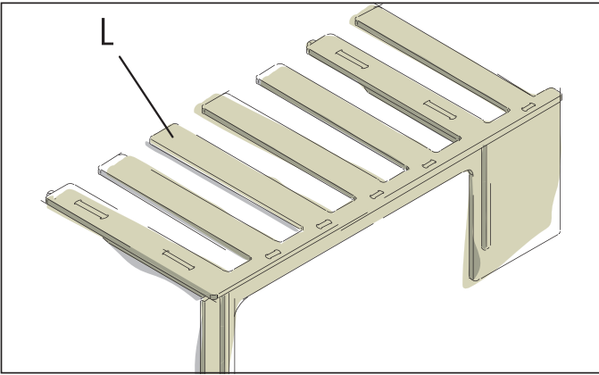
Pose le panneau de recouvrement à lattes (L) sur la partie inférieure montée précédemment. Les tenons doivent s'insérer correctement dans les rainures pré-découpées.
