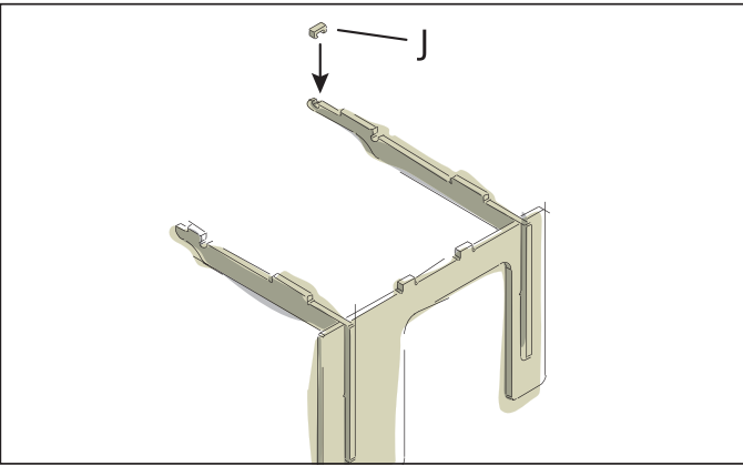
Sur le butoir (J), retire comme précédemment les petites échardes au papier abrasif. Emboîte le butoir dans la rainure arrière de l'étau coudé (H).
