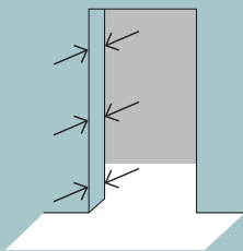
Profondeur On mesure l'épaisseur du mur fini des deux côtés de l'ouverture du mur (en tenant compte du crépi, du carrelage etc.).
