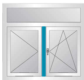
Zweiflügelige Fenster mit Dreh-Kipp-Mechanismus und beweglichen Pfosten
