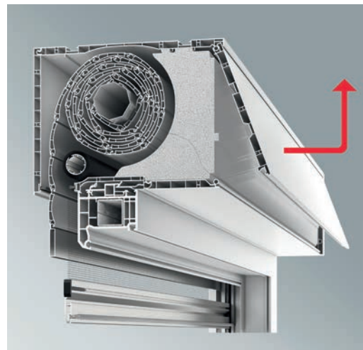
Typ A Expert XT – Revision* innen hinten Kasten innen eckig Putzträger aussen möglich
