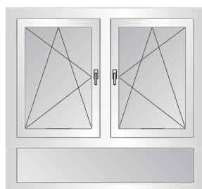
Zweiflügelige Fenster mit Dreh-Kipp-Mechanismus und beweglichen Pfosten
