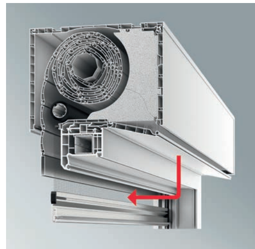
Typ A Expert XT – Revision* innen unten Kasten innen eckig Putzträger innen und aussen möglich
