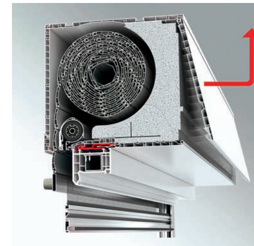
Typ A-Elite XT – Revision* innen hinten Kasten innen eckig Putzträger aussen möglich
