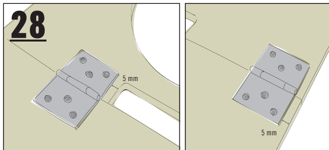
28 MONTER LES RABATS LATÉRAUX SUR LE PLAN DE TRAVAIL
