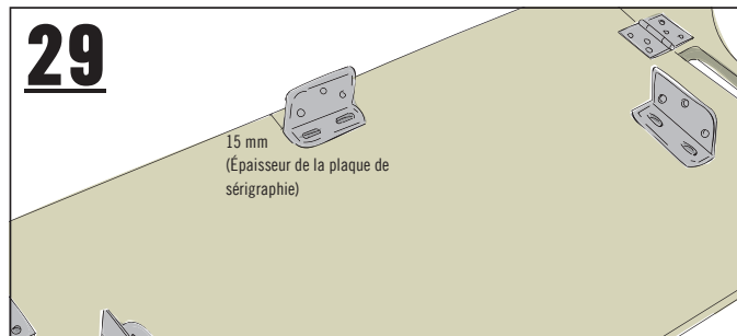
29 MONTER LES ÉQUERRES SUR LE PLAN DE TRAVAIL
