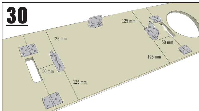
30 MONTER LES ÉQUERRES SUR LE PLAN DE TRAVAIL
