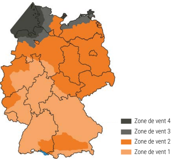
Pressions simplifiées pour les bâtiments h \leq 25 m selon DIN EN 1991-1-4/NA
