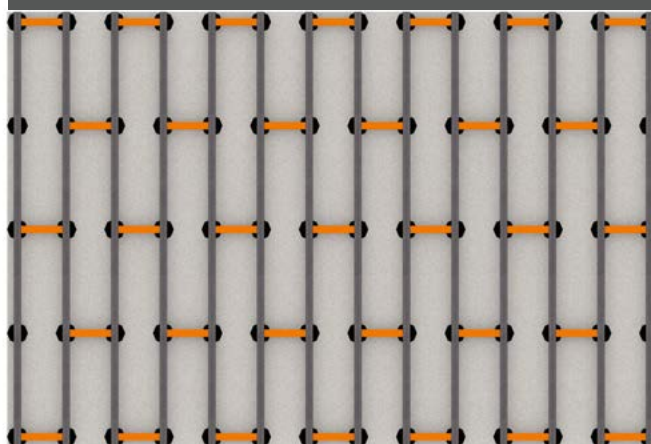
Construction avec renfort transversal
