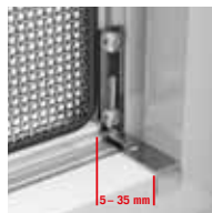
Pattes d'accrochage réglables en hauteur
