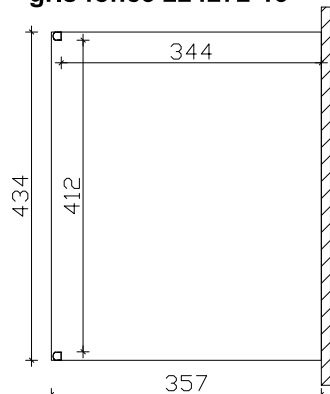
Plan au sol
