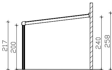
Coupe
