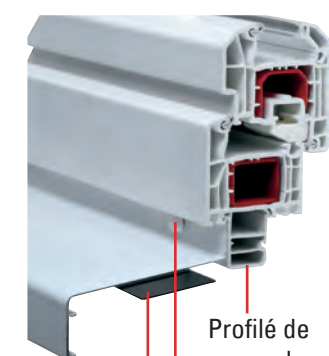
Vis pour rebords de fenêtre avec capuchon
