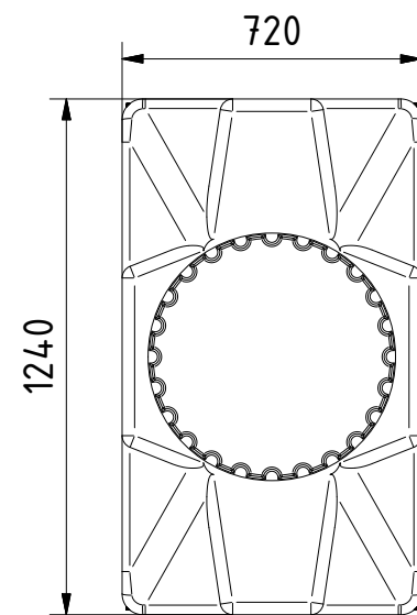
Ansicht von oben vue du dessus
