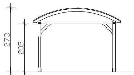
Ansicht Front
