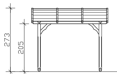
Ansicht Seite
