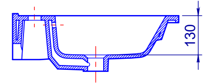
A-A KESİTİ
