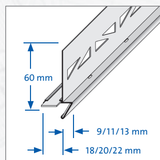
Angle extérieur vertical
