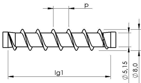
Filetage secondaire
