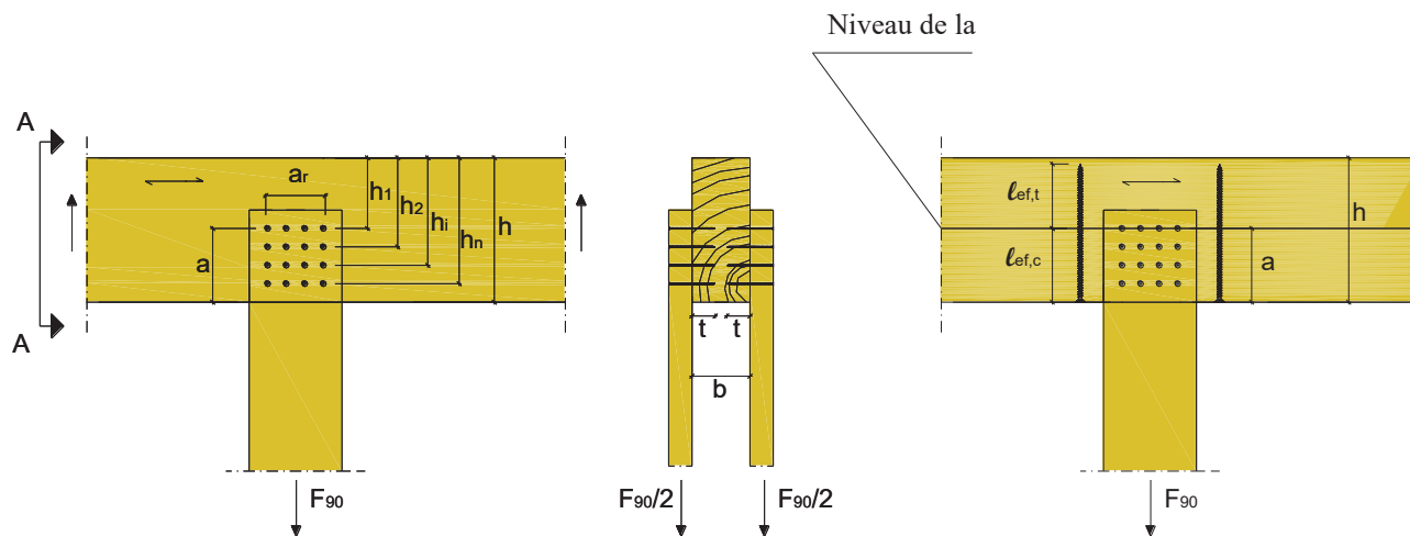
Figure 5 : Exemple de renforcement en traction d'un effort d'assemblage perpendiculaire au fil
