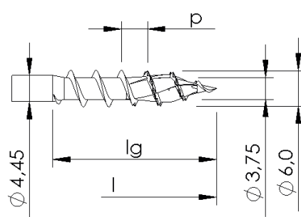
Sans variation de filetage, avec pointe nervurée et nervures de fraisage
