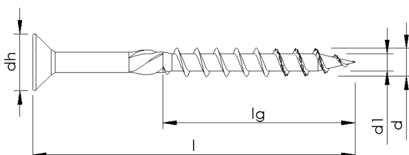
Filetage partiel sans variation, avec nervures de tige et pointe nervurée
