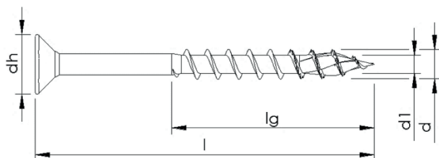
Filetage partiel sans variation, sans nervures de tige, avec pointe nervurée et nervures de fraisage
