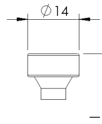
Tête cylindrique avec Fraisage
