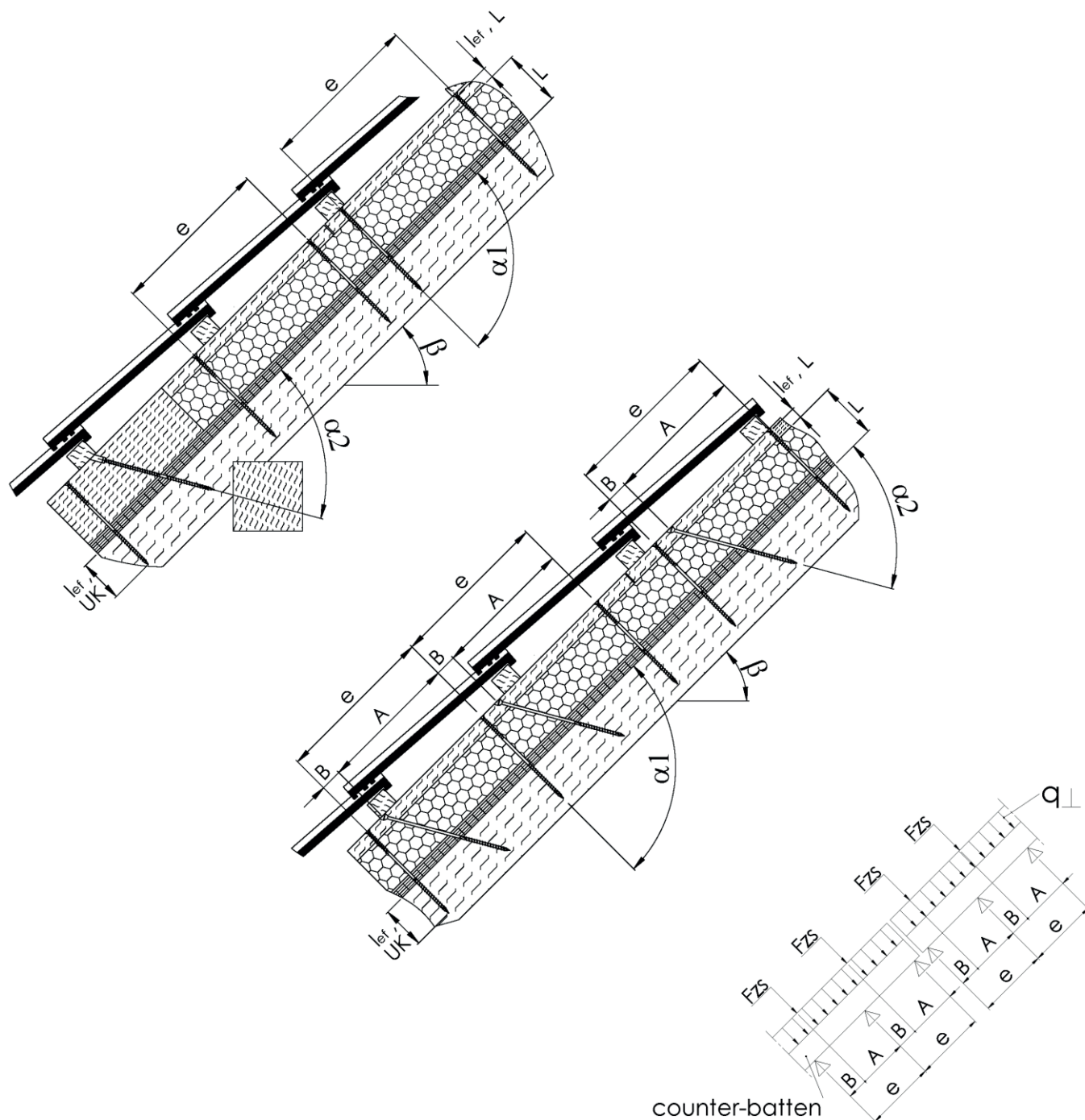
Figure 8 Mise en œuvre d'un isolant thermique sur des chevrons - système structural pour des vis inclinées alternativement et une poutre continu sous charges linéaires constantes provenant des actions exercées sur le plan de la toiture q_{\perp} et des charges concentrées provenant des vis en traction F_{ZS}
