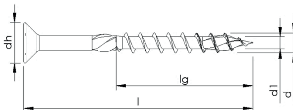
Filetage partiel sans variation, avec nervures de tige, avec pointe nervurée et nervures de fraisage
