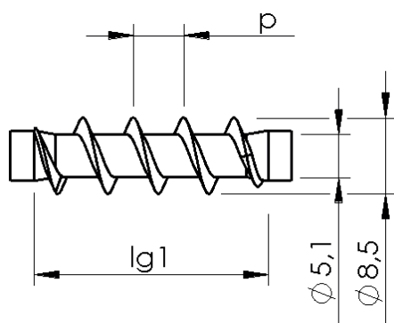
Filetage secondaire
