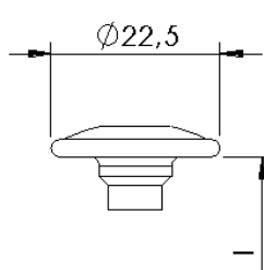
Tête bombée à embase cylindrique
