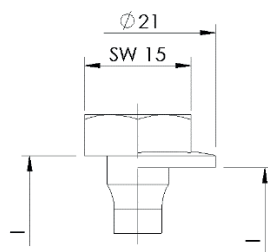
Tête hexagonale avec ou sans rondelle
