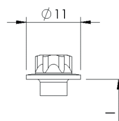
Tête hexagonale externe avec ou sans rondelle
