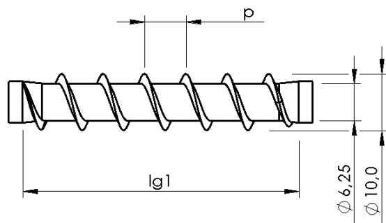
Filetage secondaire
