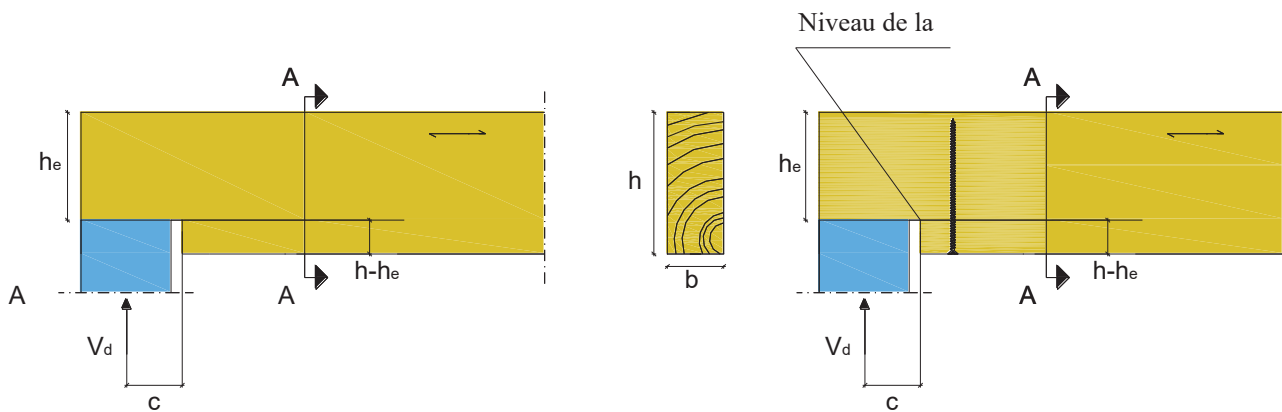
Figure 6 : Exemple de renforcement en traction d'un appui de poutre entaillé
