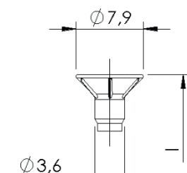
Tête plate fraisée 90° avec perçage central, avec ou sans nervures de fraisage
