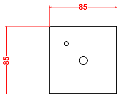
VISTA SUPERIORE
