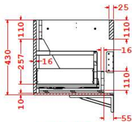
SEZIONE A-A
