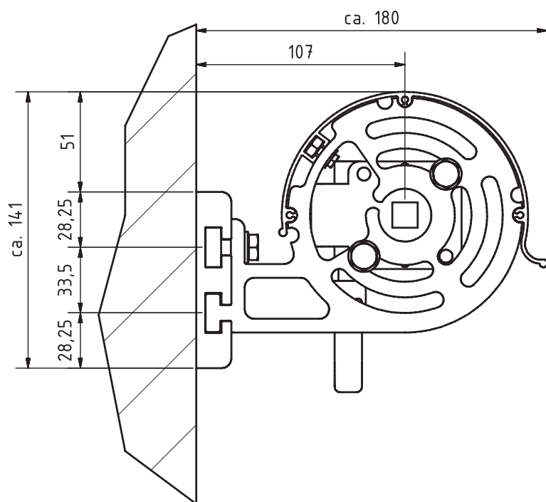
Vue de côté store de façade Type A et Type S
