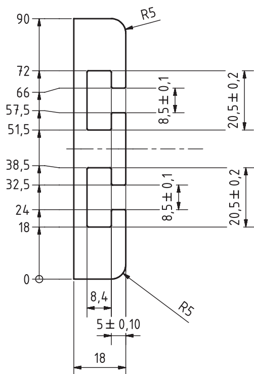
Console pour montage mural Type A et Type S
