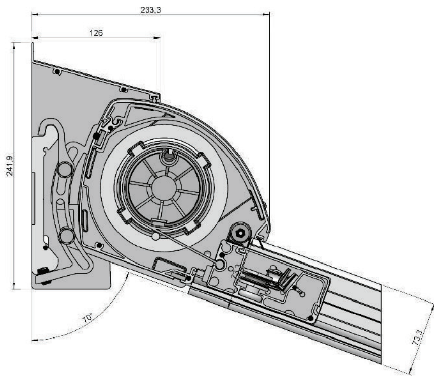
Vue de côté montage mural en mm
