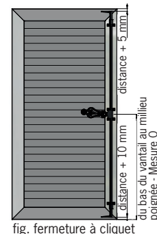
fig. fermeture à cliquet
