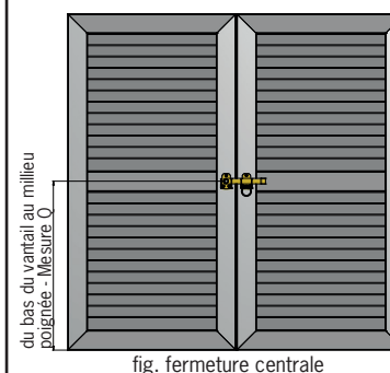
fig. fermeture centrale
