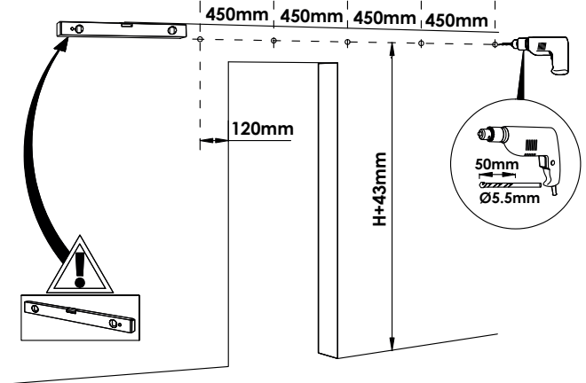
2B Montage op houten muur - Wand aus Holz Wooden wall - Mur à bois
