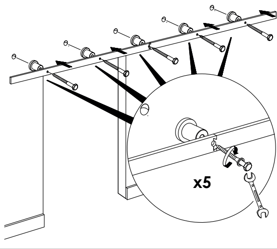
2B Montage op houten muur - Wand aus Holz Wooden wall - Mur à bois
