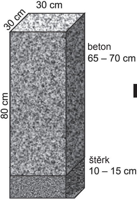
ZÁKLADY
