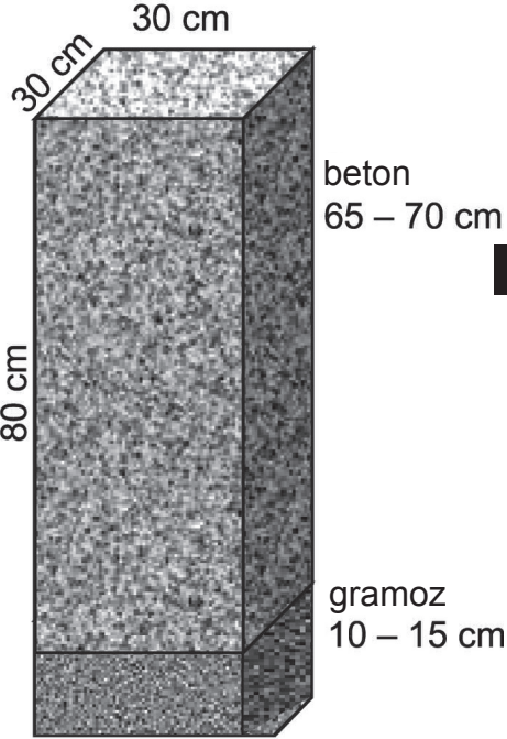
TEMELJ
