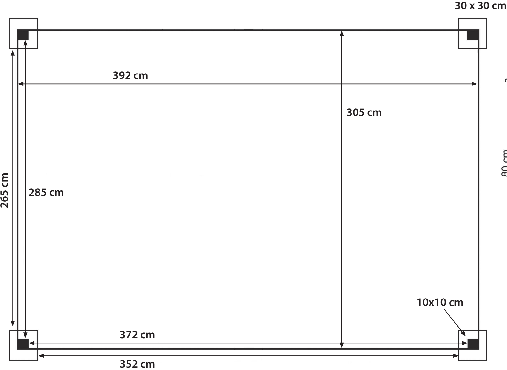
FUNDAMENT
