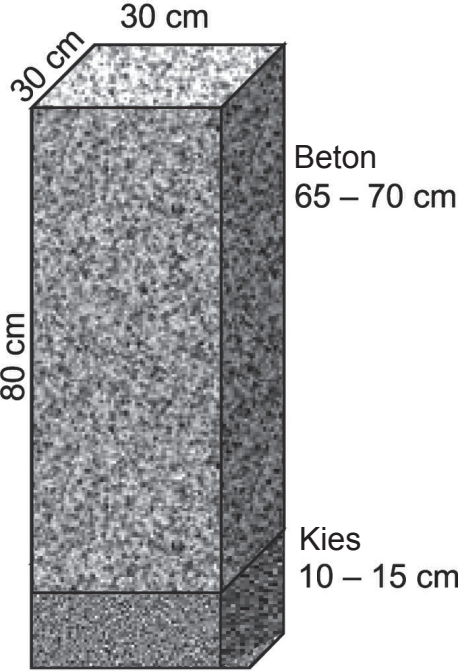
FUNDAMENT
