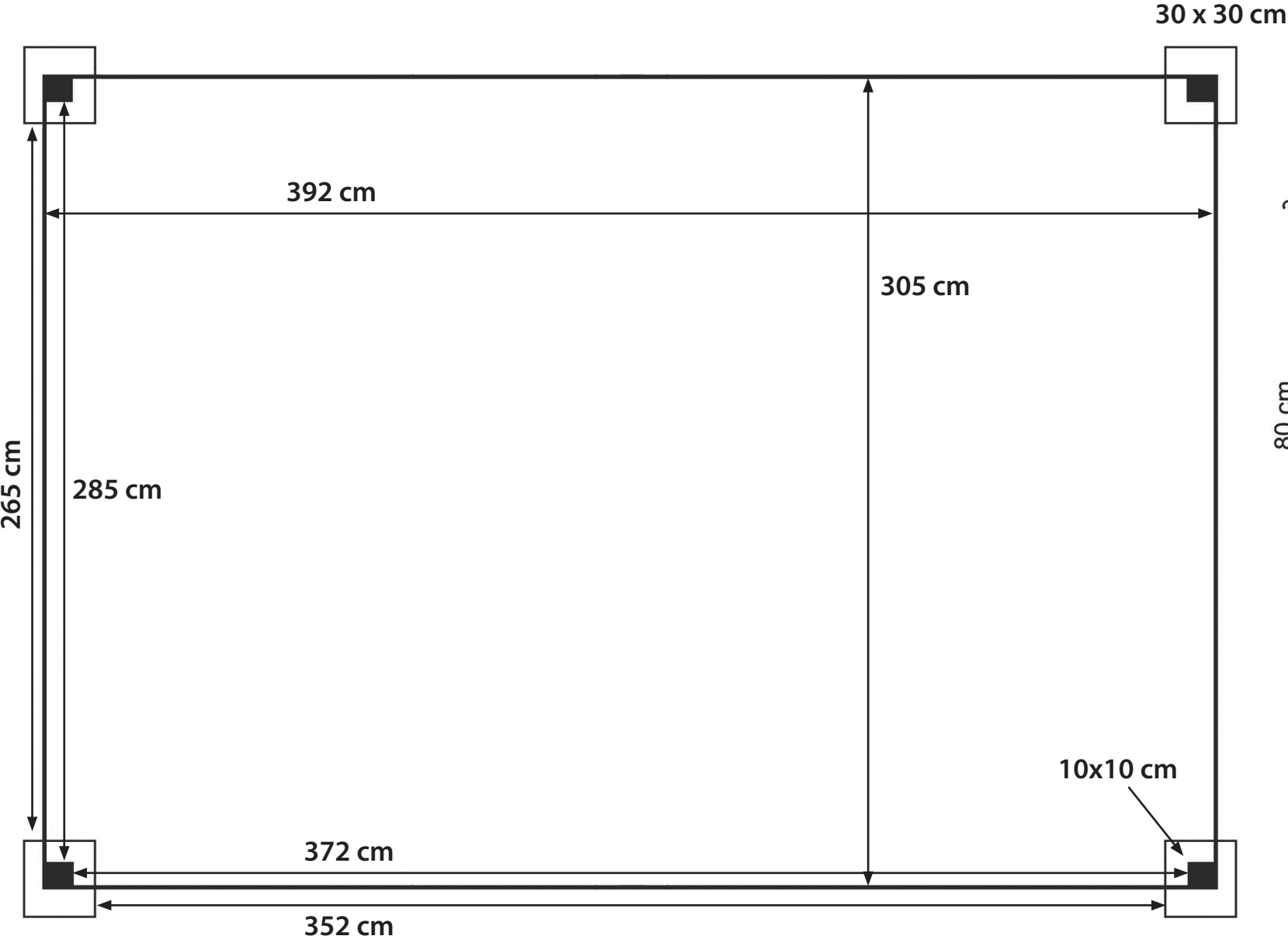
FUNDAMENT
