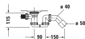
Siphon für Whirlwanne # 760449
