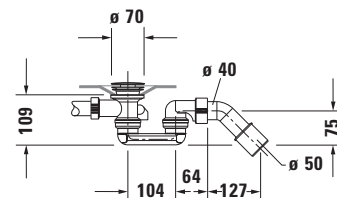
Siphon für Badewanne # 700453
