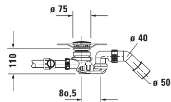
Siphon mit Bodenzulauf für Whirlwanne # 760450
