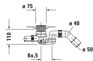
Siphon mit Bodenzulauf für Badewanne # 700449
