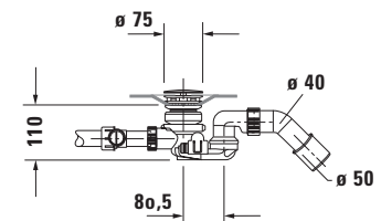
Siphon mit Bodenzulauf für Whirlwanne # 760451
