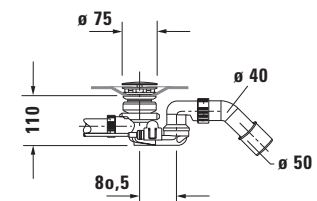
Siphon mit Bodenzulauf für Badewanne # 700451
