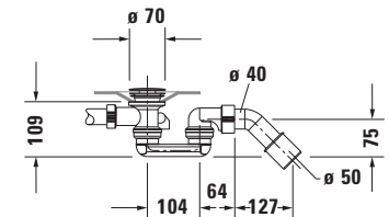
Siphon für Badewanne # 700451
