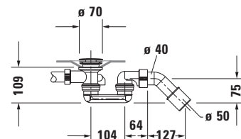
Siphon für Badewanne # 700450
