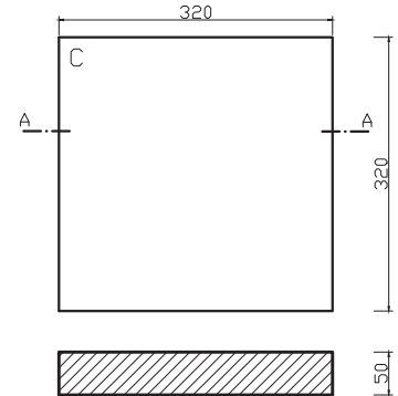
Querschnitt A-A
