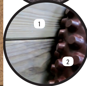
1- Ossature composite 2- Rouleau de protection et de drainage alvéolaire en PEHD
