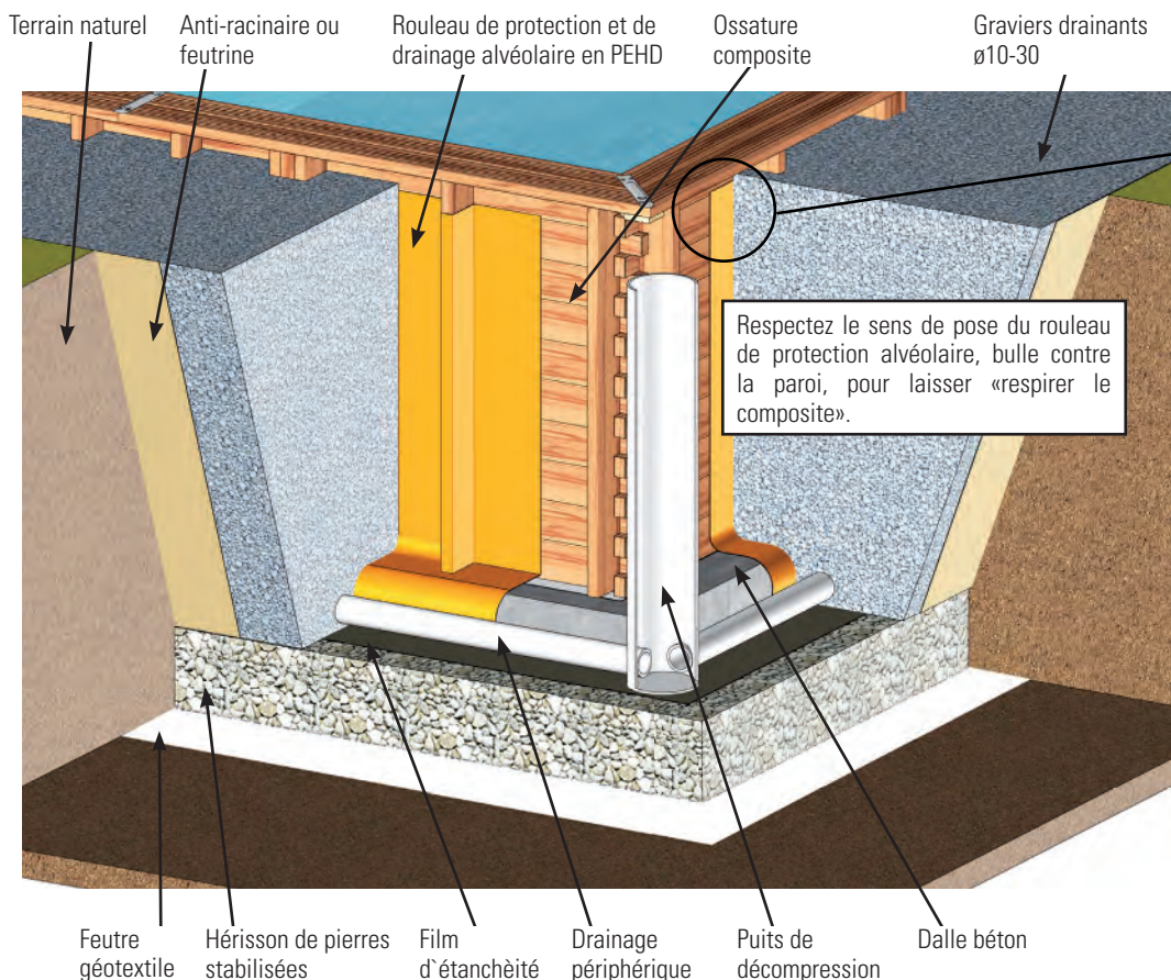
1- Ossature composite 2- Rouleau de protection et de drainage alvéolaire en PEHD
