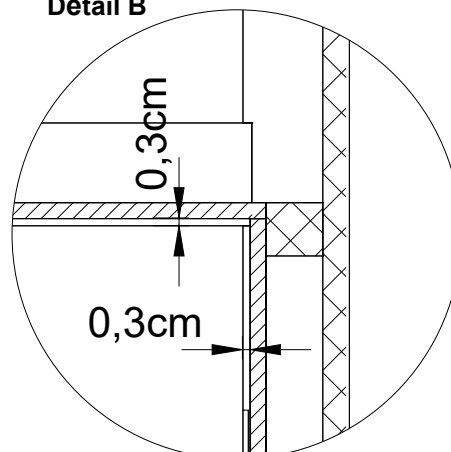
Détail B
