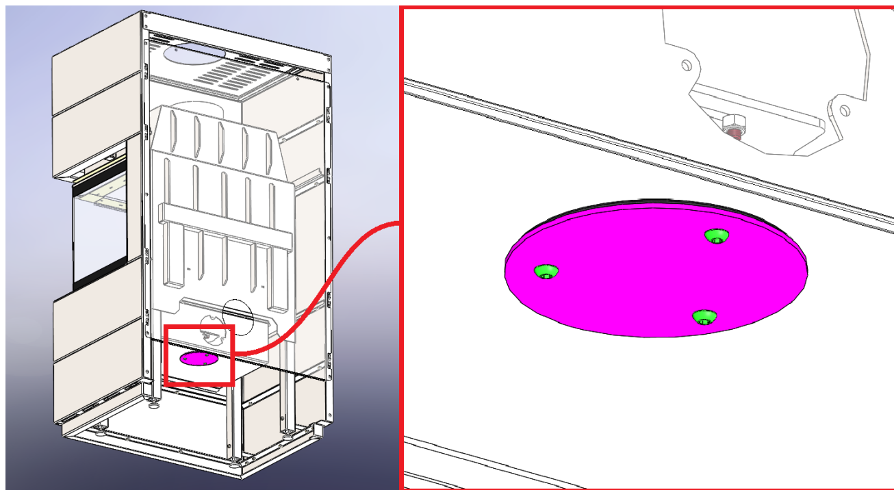
Figura 3 Poziționarea capacului
