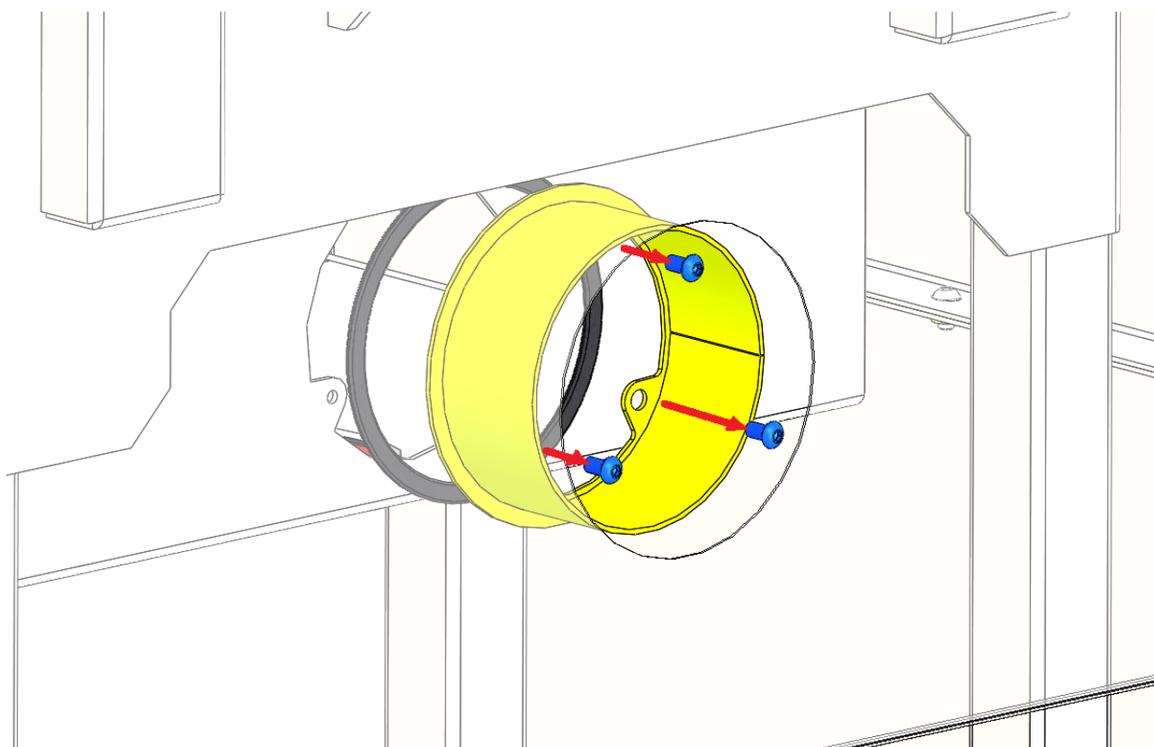
Obrázek 6 Odstranění připojení pro externí přívod vzduchu
