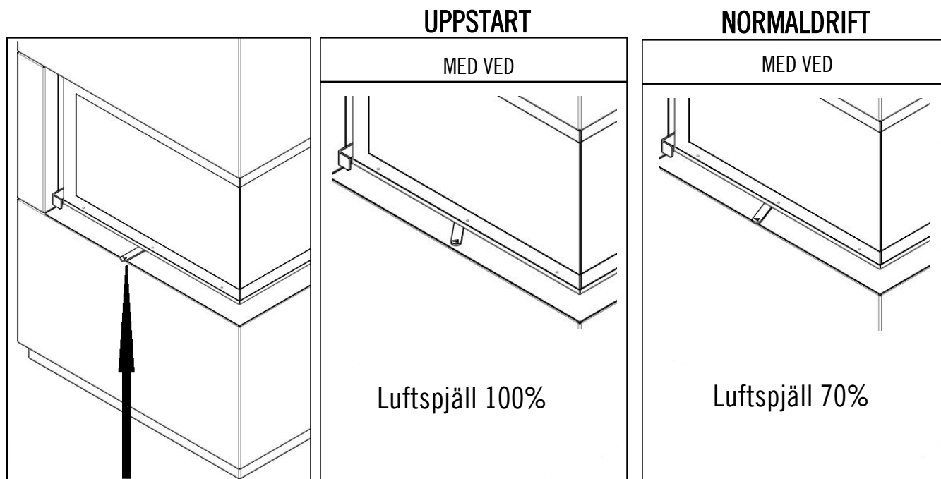
Luftspjäll
