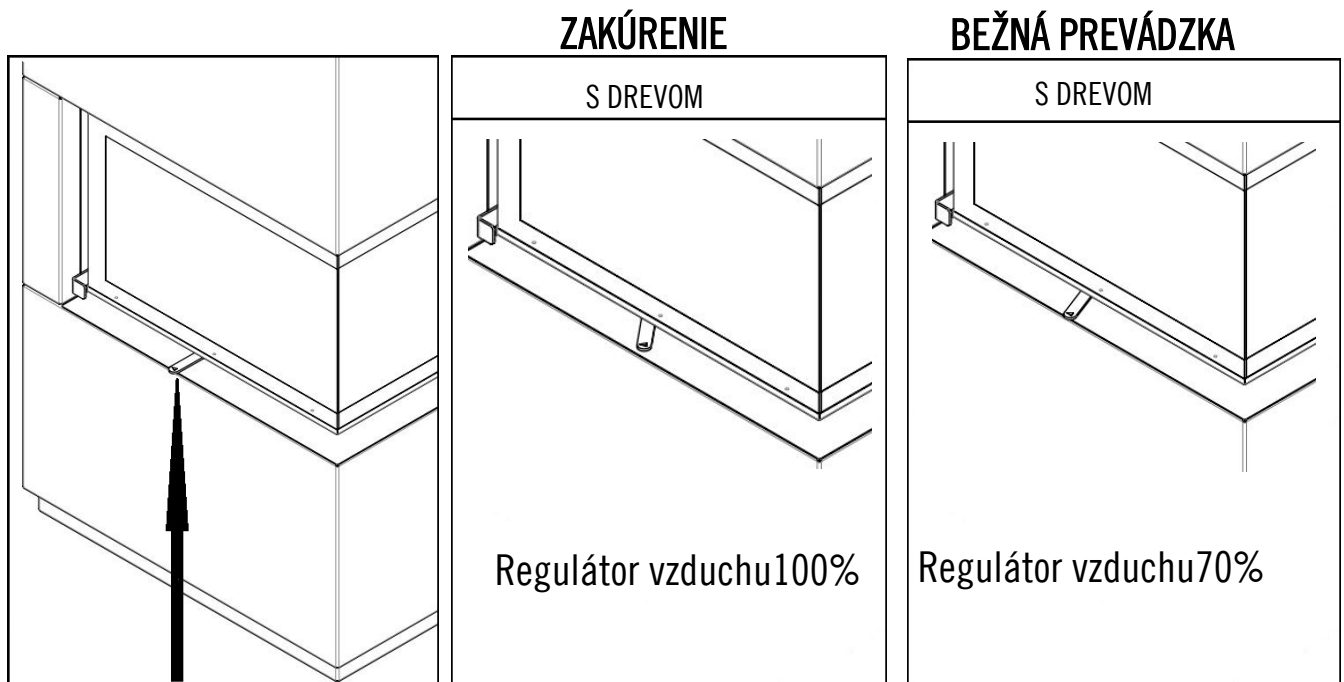
Regulátor vzduchu
