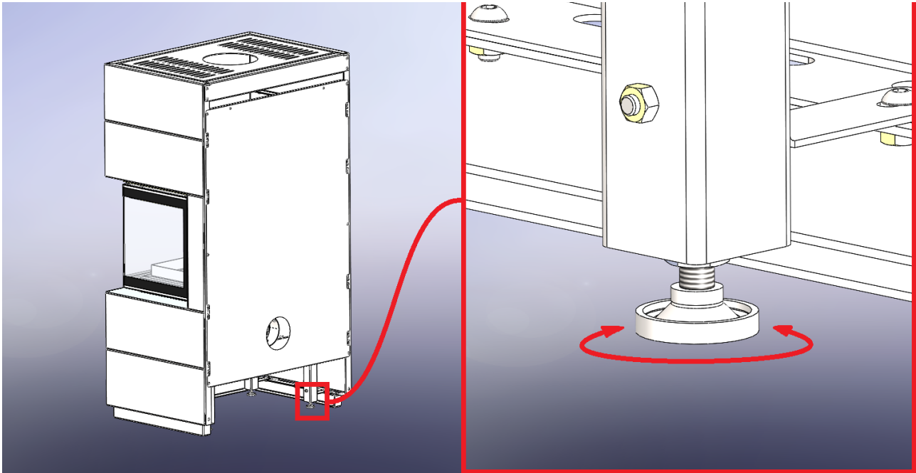
Abbildung Die Höhe des Kamins einstellen, in eine waagerechte Position bringen
