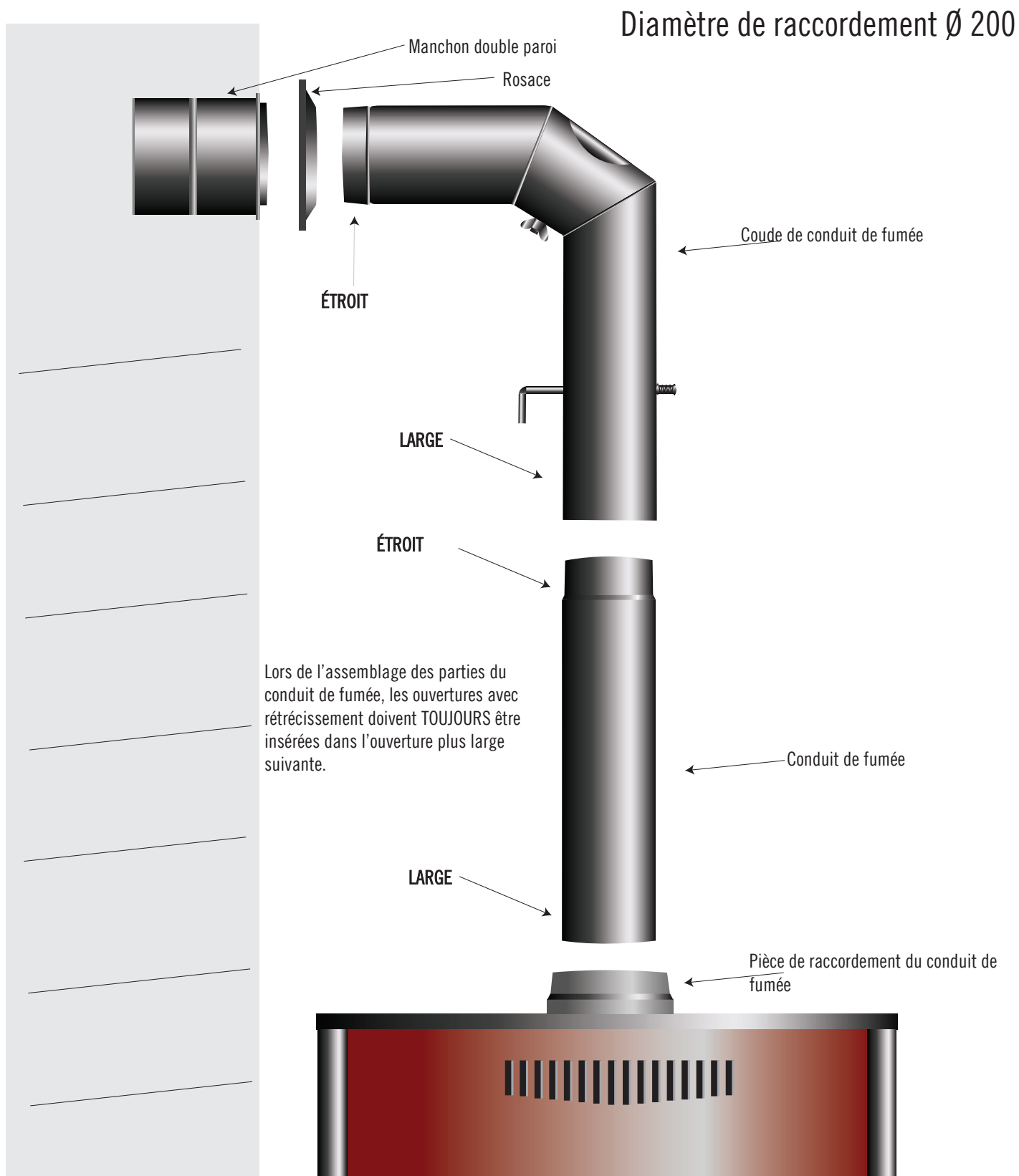
Figurel : Raccordement du poêle à bois à la cheminée
