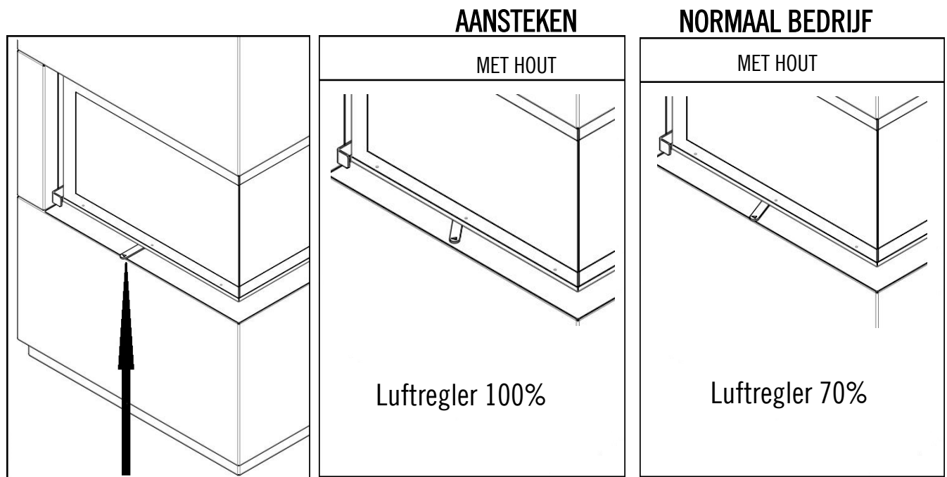
Luchtregler
