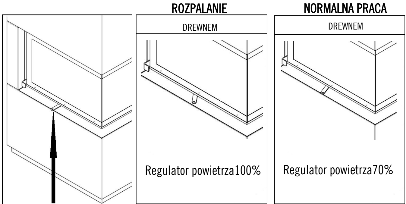
Regulator powietrza
