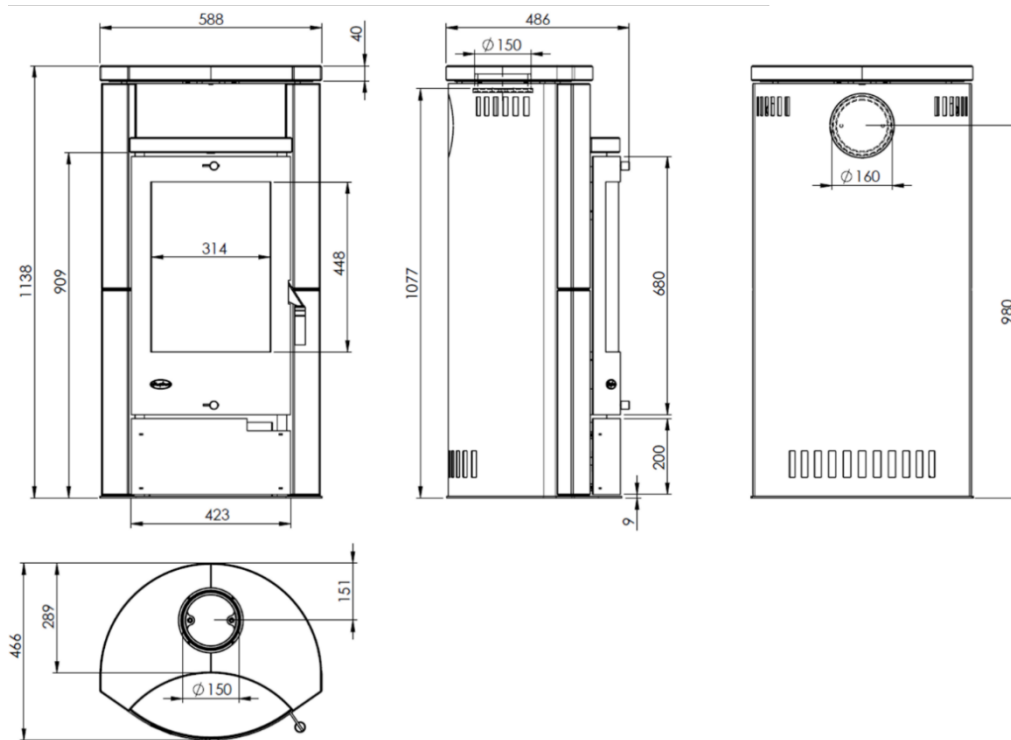
Abbildung 2 - Hauptmaße
