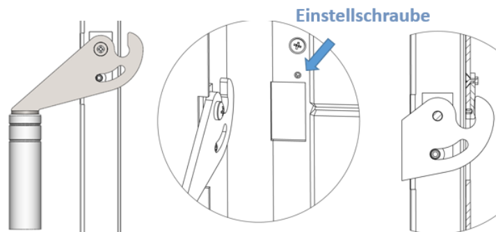
Abbildung 12 - Verriegelung
