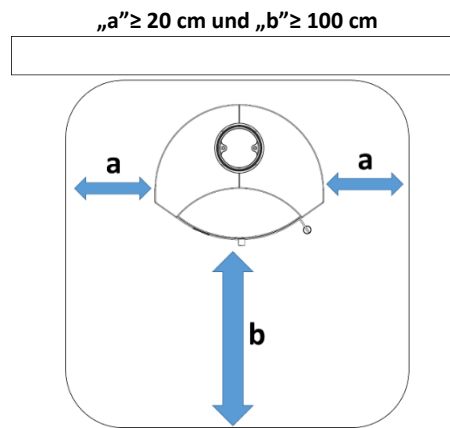
Abbildung 5 - Bodenplatte
