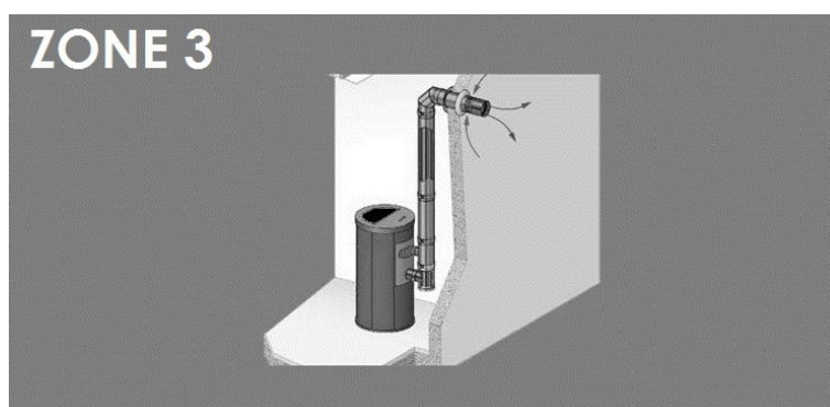
Fig. 10 - Schéma de principe du système concentrique avec terminal horizontal (ZONE 3)
