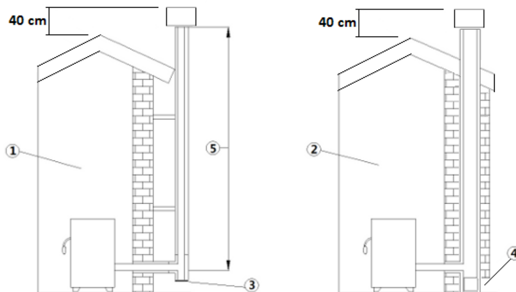
Fig. 2 - Conduit des fumées
