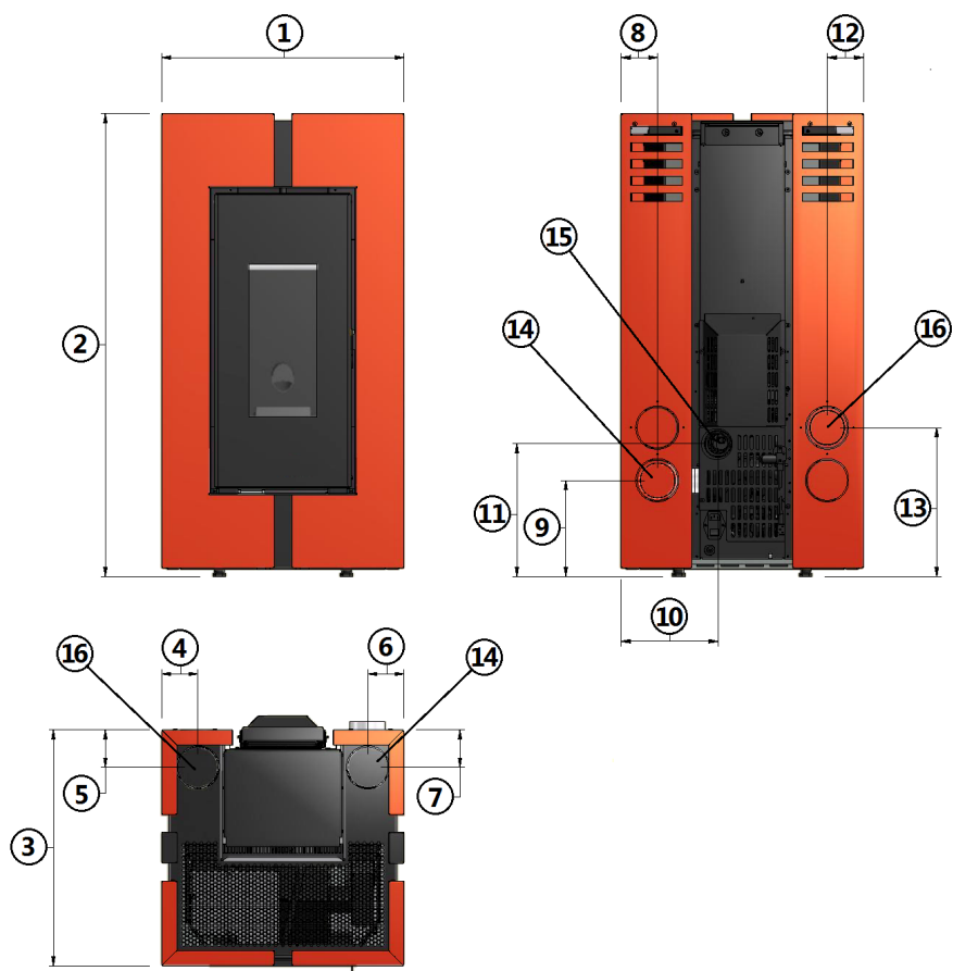
Fig. 20 - Dimensions générales: Doge³ Plus
