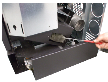
Fig. 83 - Nettoyage avec nettoie-pipes 2
