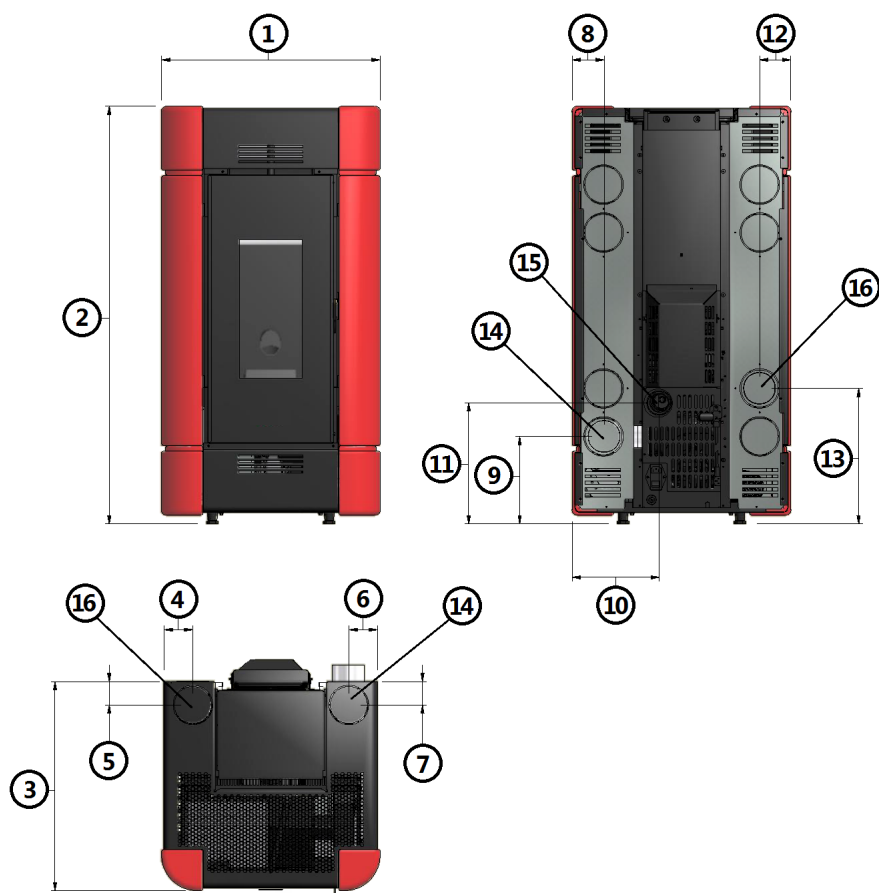
Fig. 19 - Dimensions générales: Sire³ Plus
