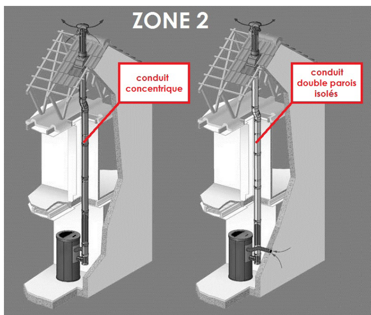
Fig. 9 - Schéma de principe du système concentrique avec terminal vertical (ZONE 2)
