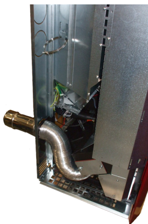
Fig. 50 - Positionnement des tubes arrière
