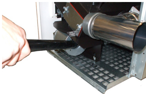
Fig. 90 - Nettoyage de le ventilateur ambiant
