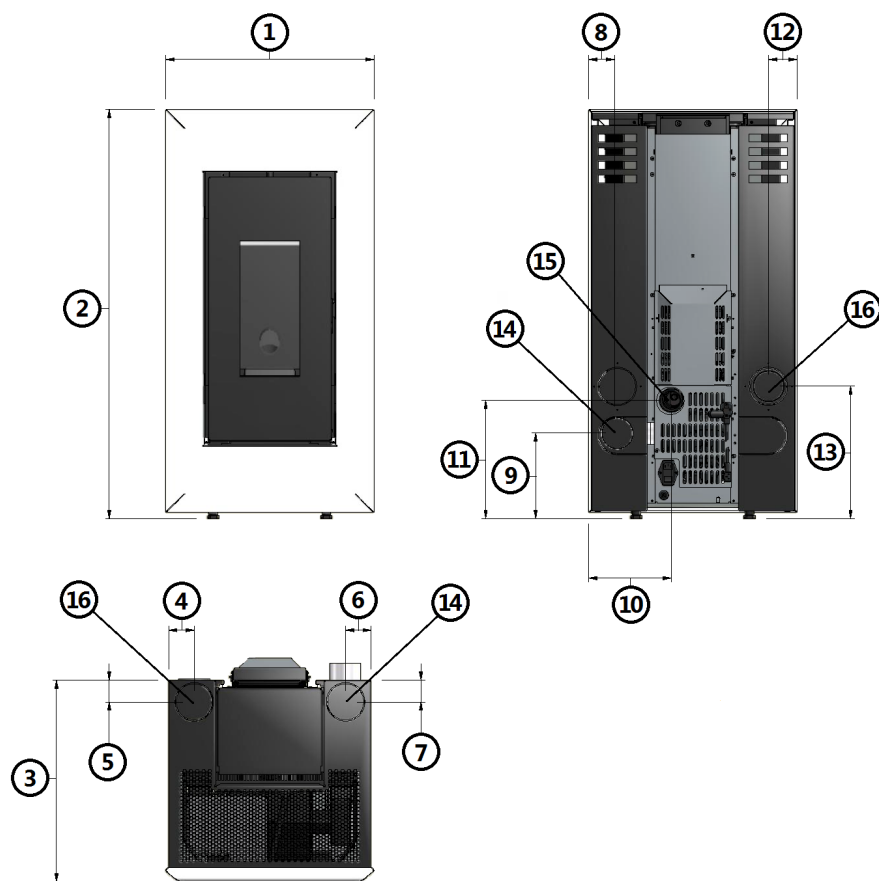
Fig. 18 - Dimensions générales: Vega / Trend
