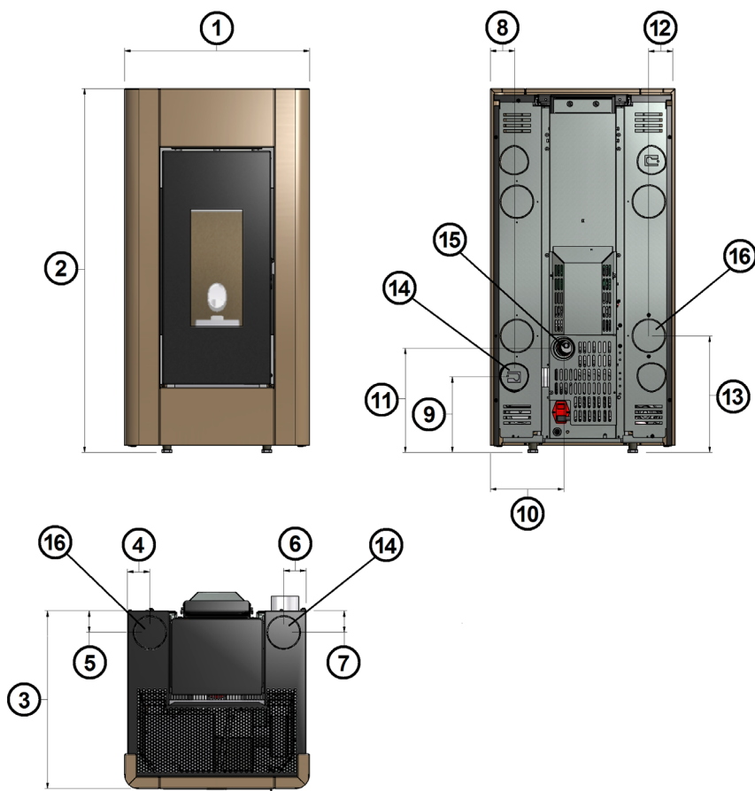
Fig. 22 - Dimensions générales: Prince³ / Prince³ Plus
