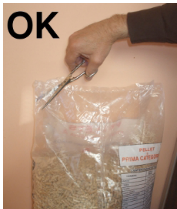
Fig. 56 - Ouverture correcte du sac des granulés
