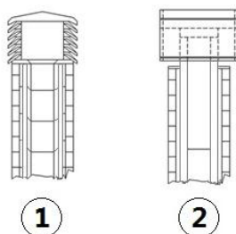
Fig. 5 - Sortie de toit
