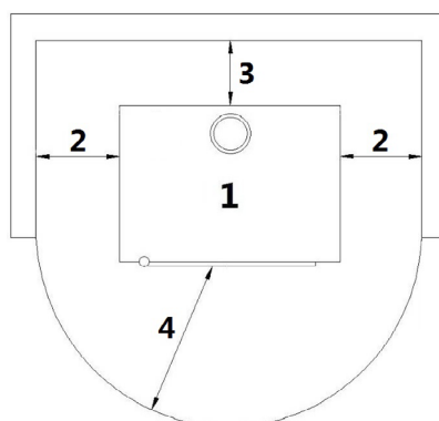
Fig. 24 - Installation générique
