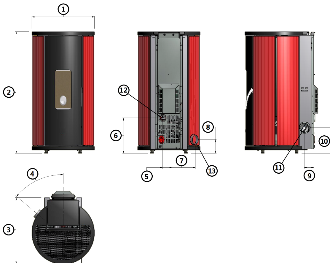
Fig. 21 - Dimensions générales: Sfera³ / Sfera³ Plus / Globe
