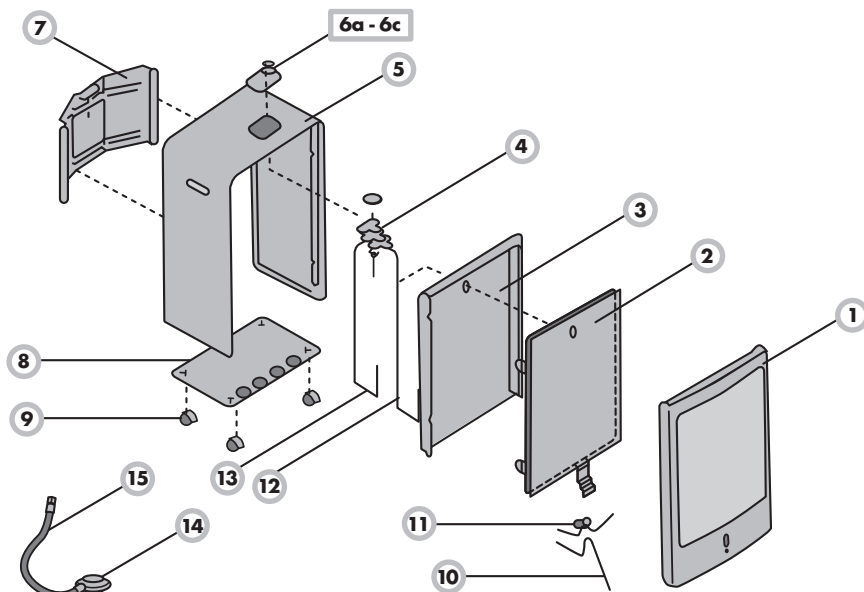
Abb. 6: Explosionszeichnung
