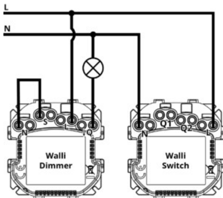
2. 2-Leiter Installation
