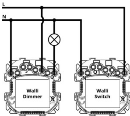
1. 3-Leiter Installation
