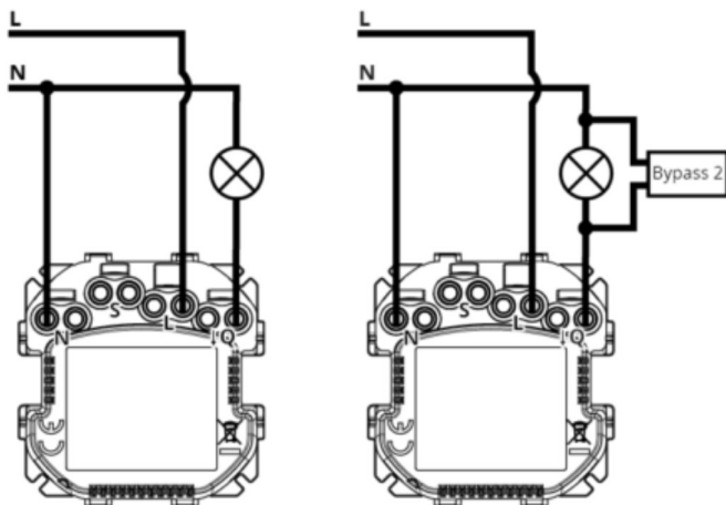
Diagramm 1: Anschlussbeispiel für 3-Leiter-Installation
