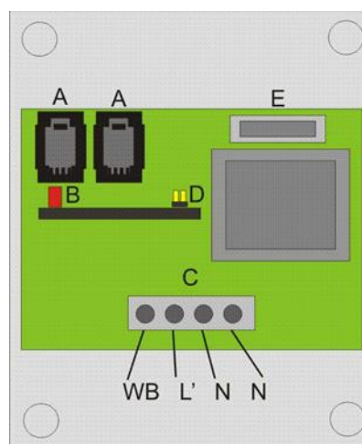
Abbildung 1 Anschlüsse
