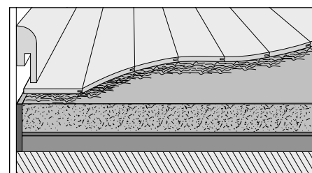
Parquet avec encollage total
