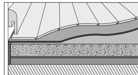
Parquet sur sous-couche Akustik-Protect 100/chape minérale
