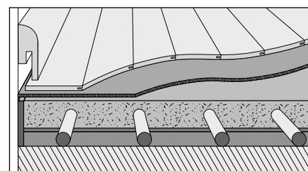
Parquet sur sous-couche Akustik-Protect avec sol chauffant à circuit d'eau chaude
