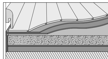
Parquet sur sous-couche Akustik-Protect/PVC/chape minérale
