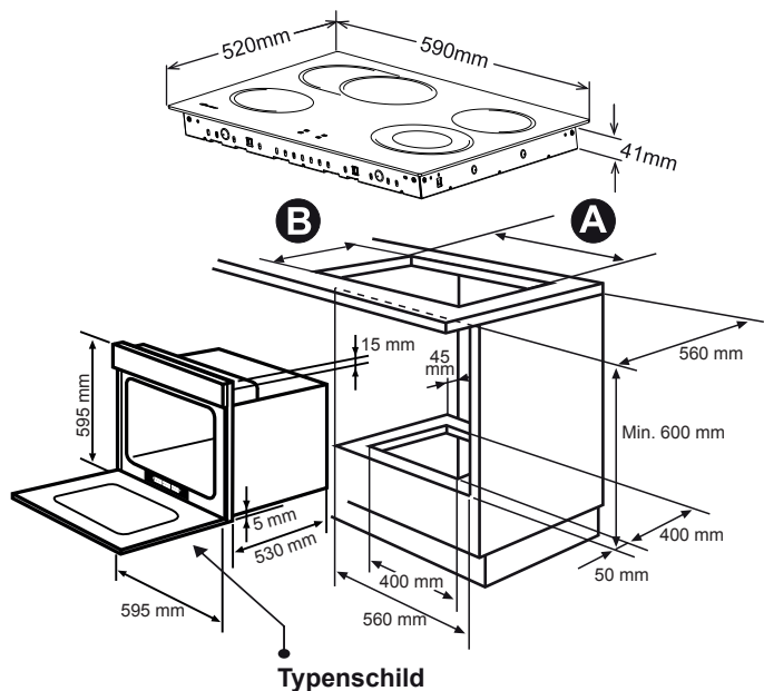
Abbildung 10 - Bündige Ofeninstallation
