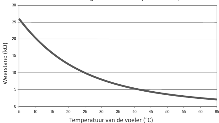
Weerstand van de regelsensor afhankelijk van de temperatuur
