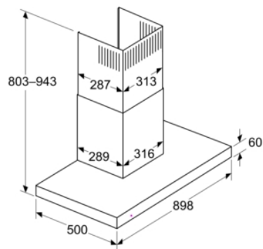
Maße in mm Ansicht Umluft
