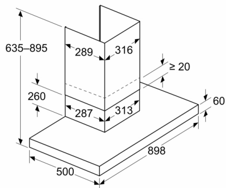
Maße in mm Gerät im Abluftbetrieb
