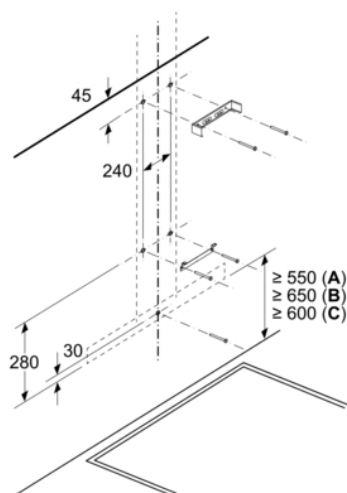
Maße in mm Wandinstallation mit Kamin
