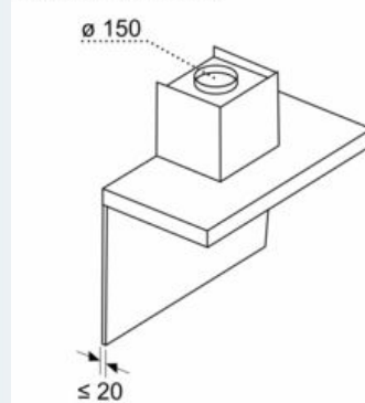
Maße in mm Wandblendentiefe
