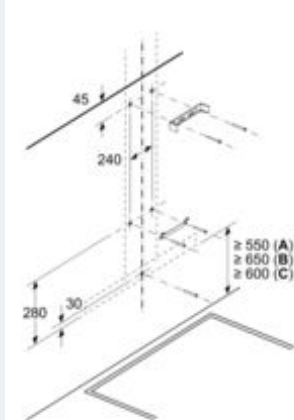
Maße in mm Wandinstallation mit Kamin
