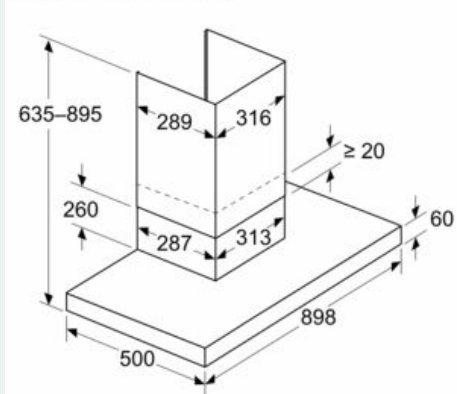
Maße in mm Gerät im Abluftbetrieb
