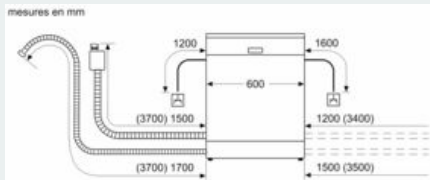
mesures en mm A prise ( ) valeurs avec kit prolongateur
