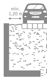
E | Verkehrs- last bis p = 5 \text{ kN/m}^2 , mit Ver- dichtungsdruck e_{vh} = 25 \text{ kN/m}^2 , Abstand: 1,2 m (bis 155 cm Höhe)/ 1,5 m (ab 180 cm Höhe) (55-105 cm Höhe ausgenommen)
