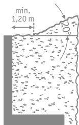
B | Böschung Geländeneigung 20^\circ , Verkehrslast bis p = 5 \text{ kN/m}^2 , Abstand: 1,2 m (bis 155 cm Höhe)/ 1,5 m (ab 180 cm Höhe)
