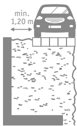
A | Verkehrs- last bis p = 5 \text{ kN/m}^2 ohne Anpralllasten, Abstand: 1,2 m (bis 155 cm Höhe)/ 1,5 m (ab 180 cm Höhe)
