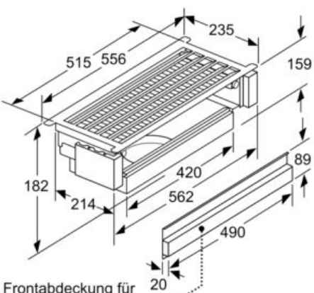
Maße in mm Montage Flachschrühhaube mit Umluftset
