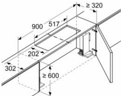
Maße in mm Montage Flachschrühhaube mit Umluftset
