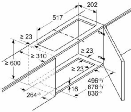
Maße in mm Montage Lüfterbaustein mit Umluftset
