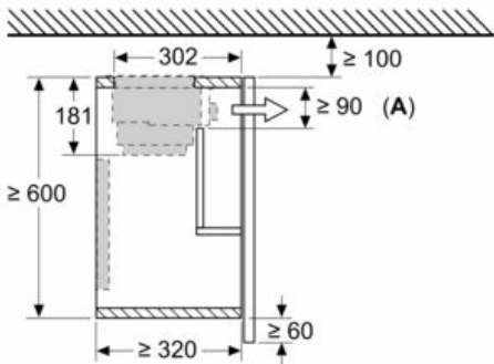
Maße in mm Montage Flachschrühhaube mit Umluftset und Absenkrahmen
