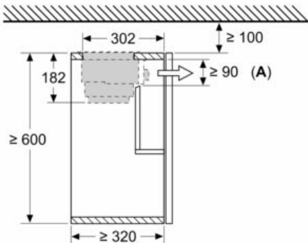
Maße in mm Montage Flachschrühhaube mit Umluftset
