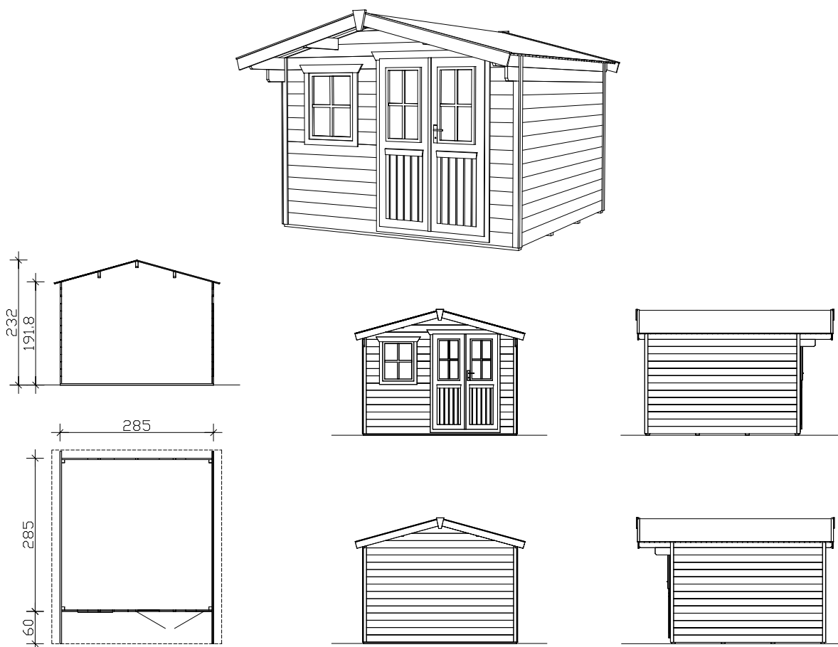
Plan, coupes et vues M 1:100
