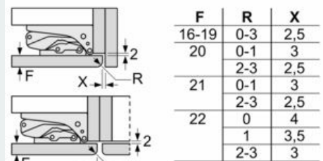
Masse in mm Empfehlung Spaltmasse für Flachscharnier
