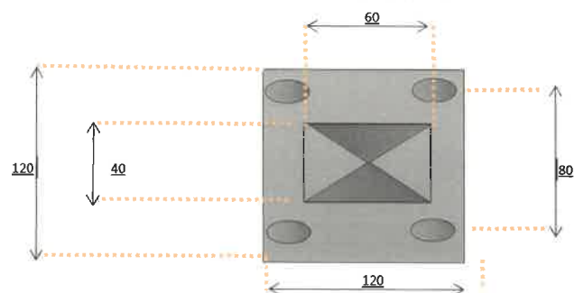
Bodenplatte 120x120 mm mit 4x Langloch 25/13
