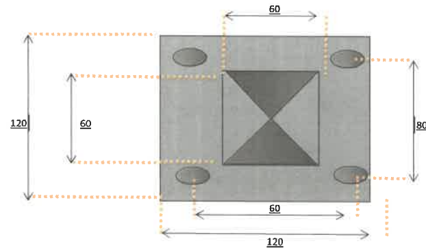
Bodenplatte 120x120mm mit 4x Langloch 25/13
